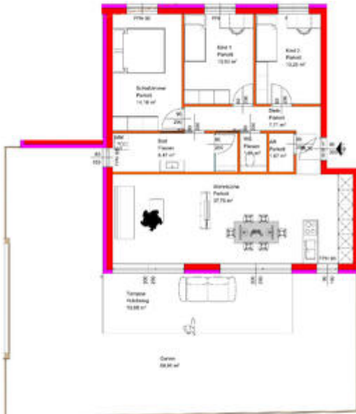
Wohnungsplan Top 1
